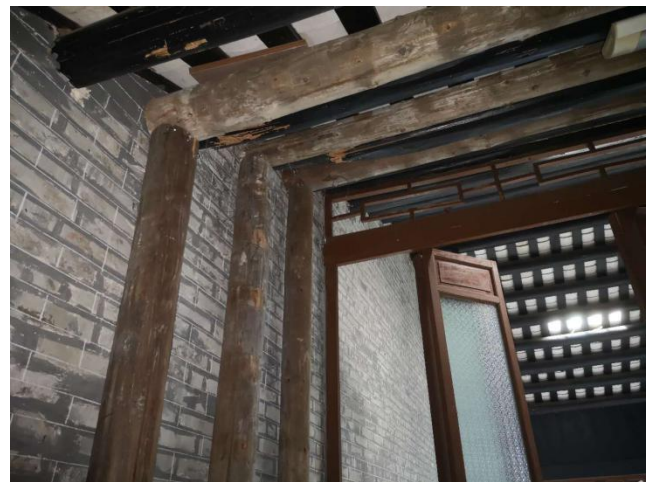
增加横梁支撑的阁楼区域
